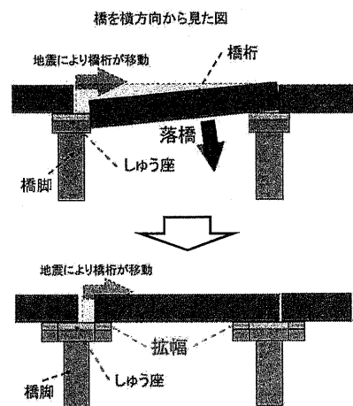
落橋防止工による橋梁の耐震対策
