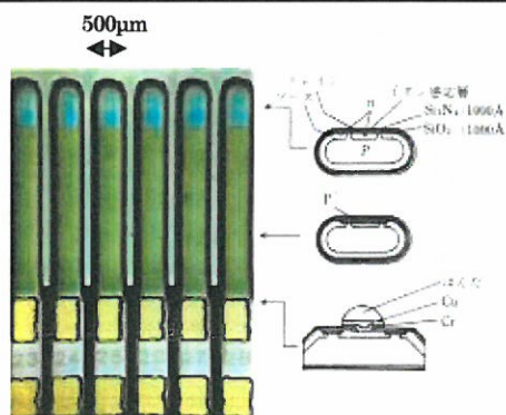
ウェハ上の半導体イオンセンサ ISFET の写真と断面構造
